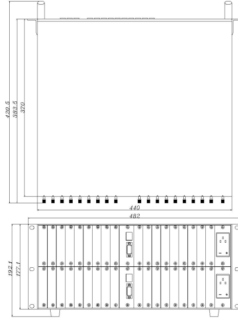
FLEX 18(MINI)
